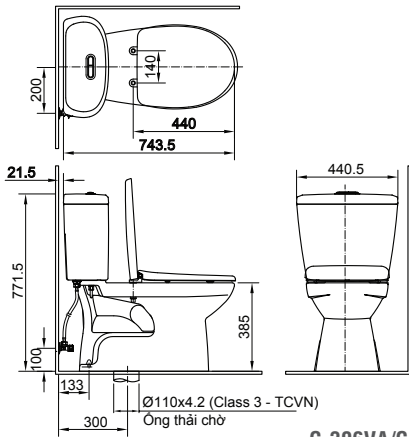
C-306VA/C-306VAN
